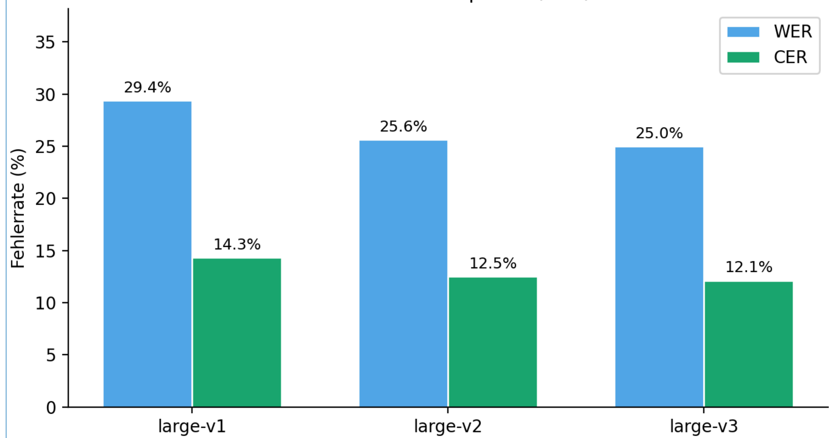
WER vs CER – Whisper v1 / v2 / v3
